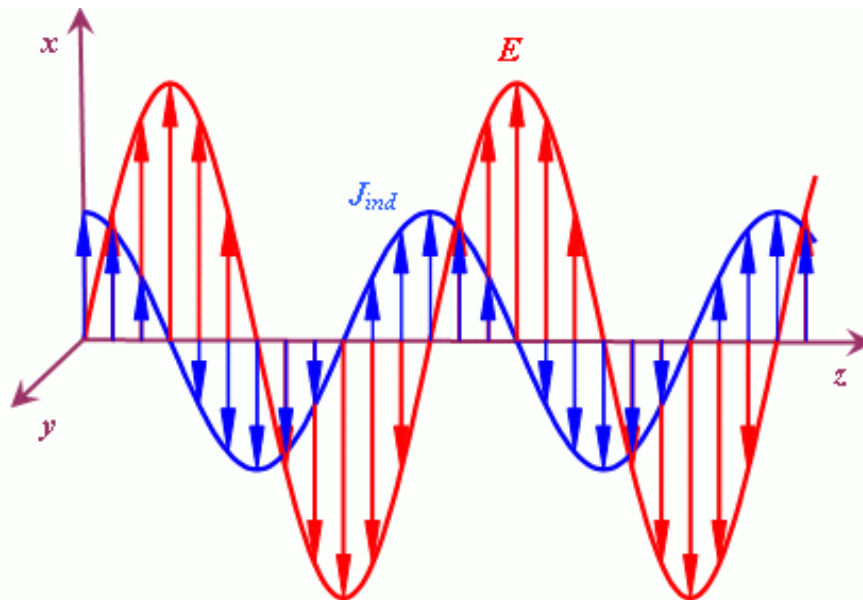
Рис. 1. Структура ЭМ волны
