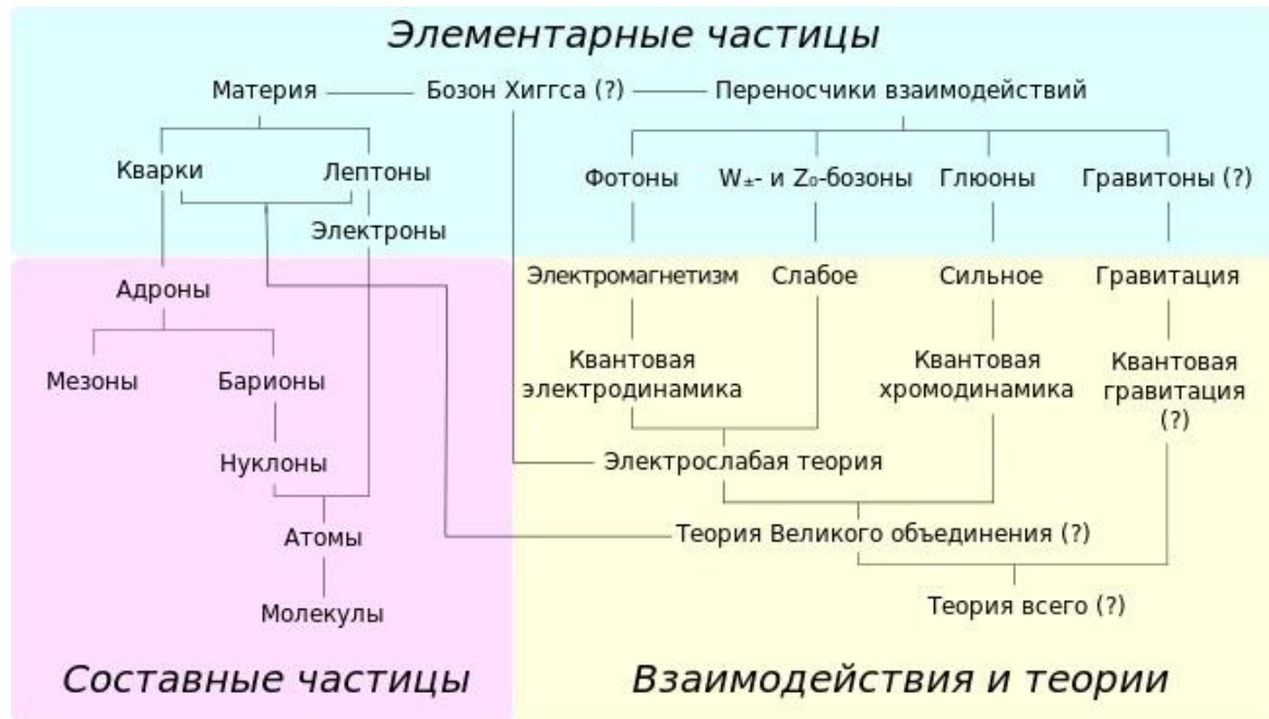
Рис. 2 Классификация элементарных частиц
